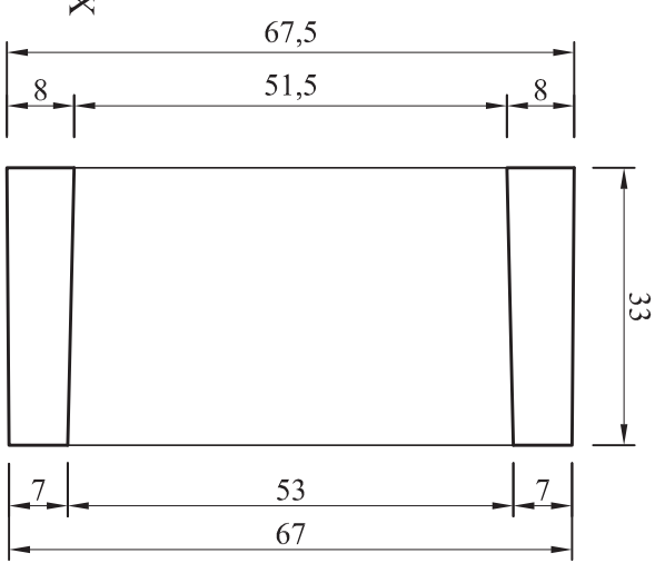
SEZIONE Y - Y
