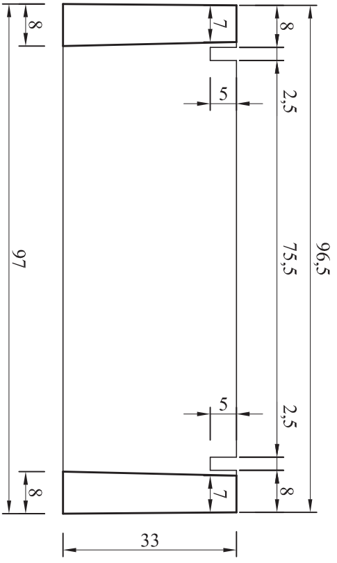
SEZIONE X - X
